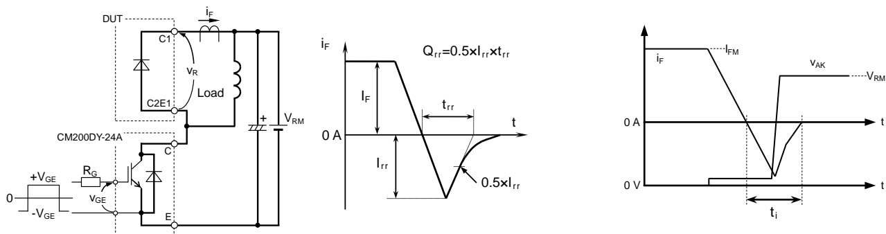
逆回復特性試験回路及び試験波形
