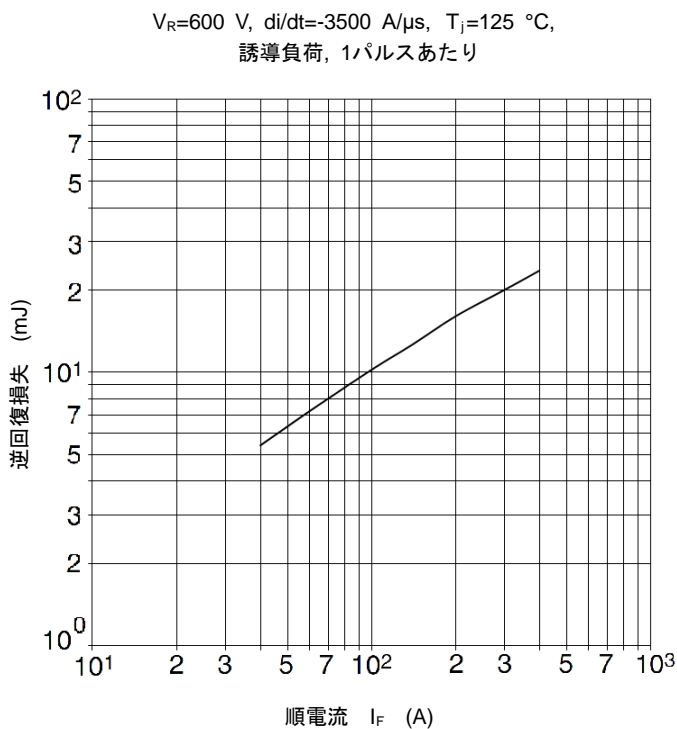
逆回復特性 (代表例)
