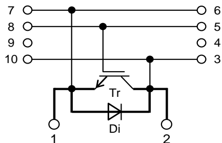
内部接続図
