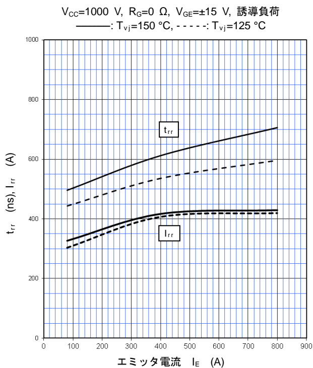
フリーホイールダイオード回復特性 (代表例)
