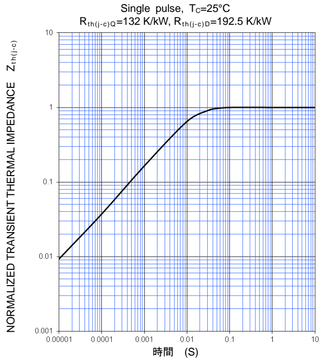
過渡熱インピーダンス特性 (最大)
