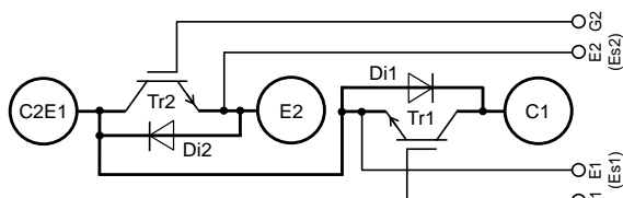
内部接続図
