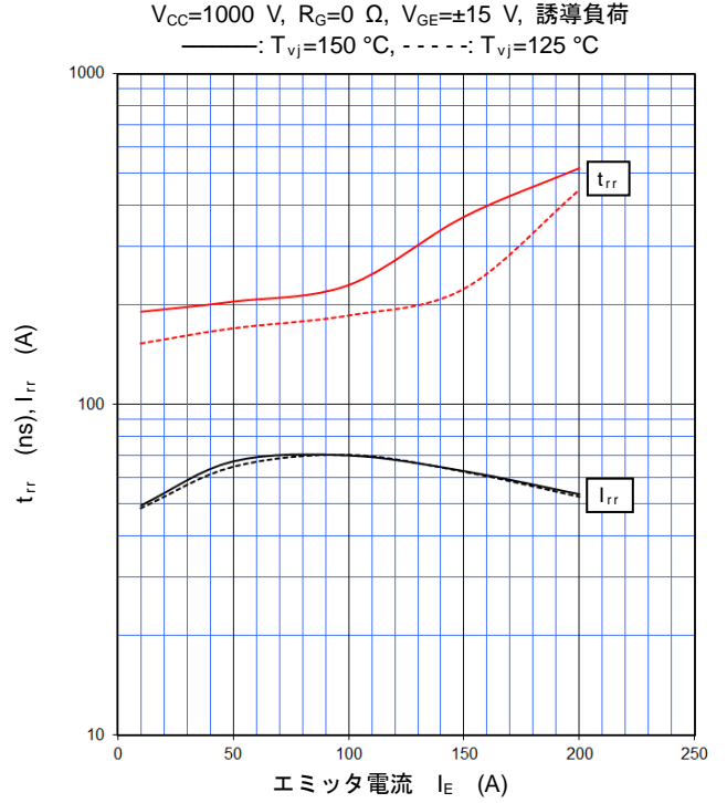
フリーホイールダイオード回復特性 (代表例)
