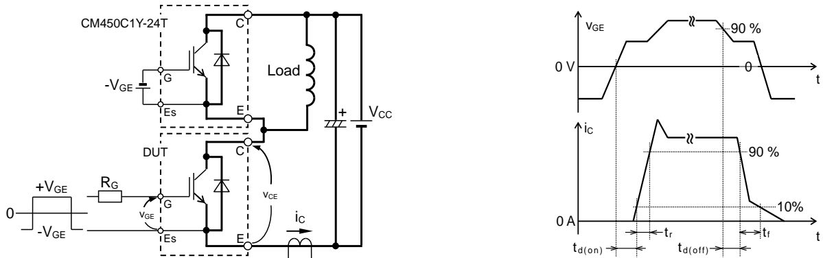
スイッチング特性試験回路及び試験波形
