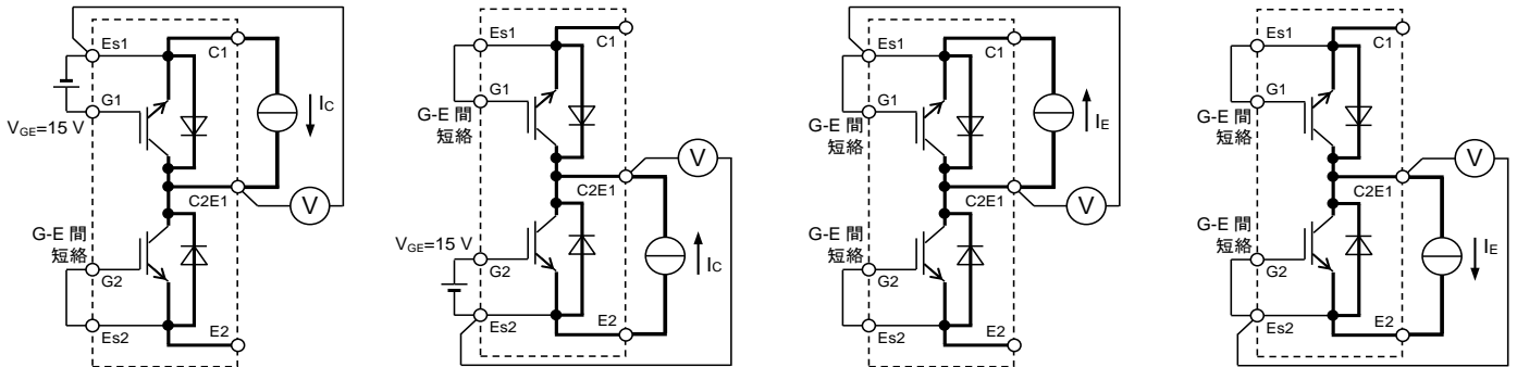
V_{CEsat} 試験回路
