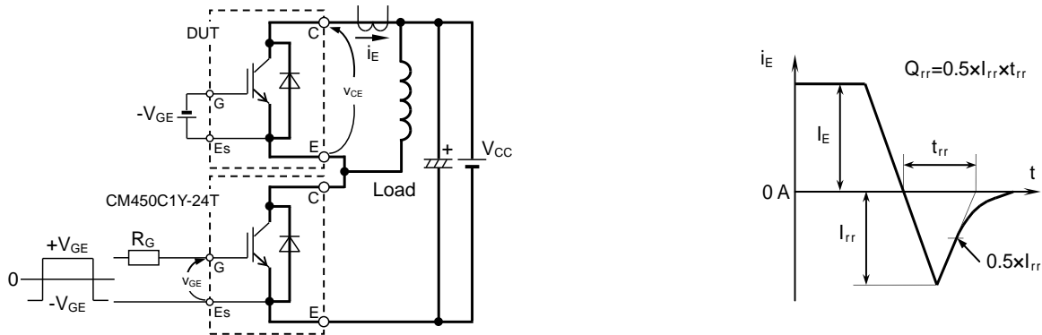
逆回復特性試験回路及び試験波形
