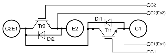
内部接続図
