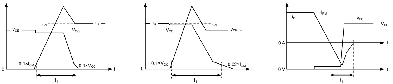
スイッチング損失及び逆回復損失試験波形（積分時間説明図）
