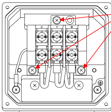
図 1 端子箱構造図
