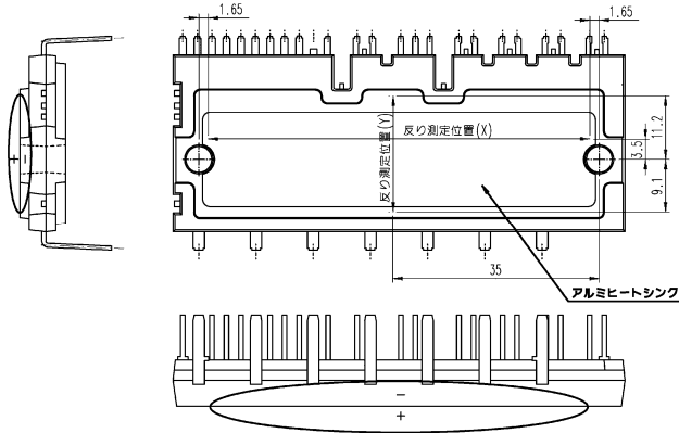
注6. 放熱面平面度測定位置
